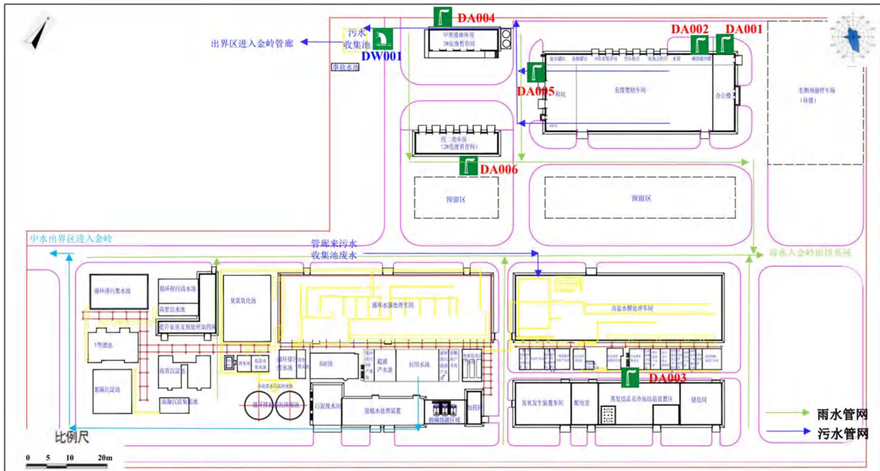
图 4.3-2 项目平面布置图
