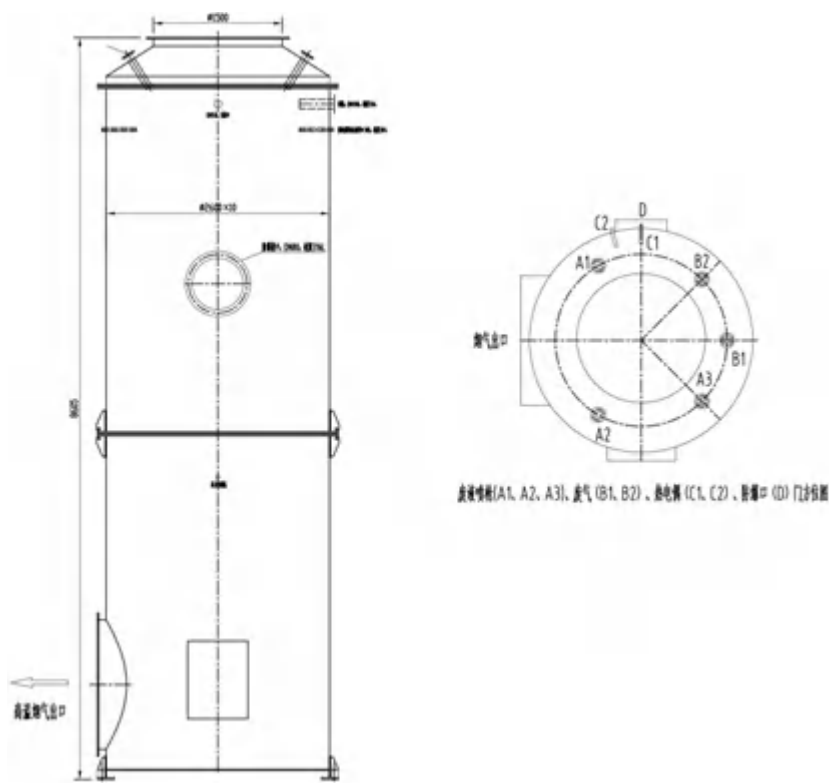
图 4.9-3 高氯焚烧炉内部结构图
