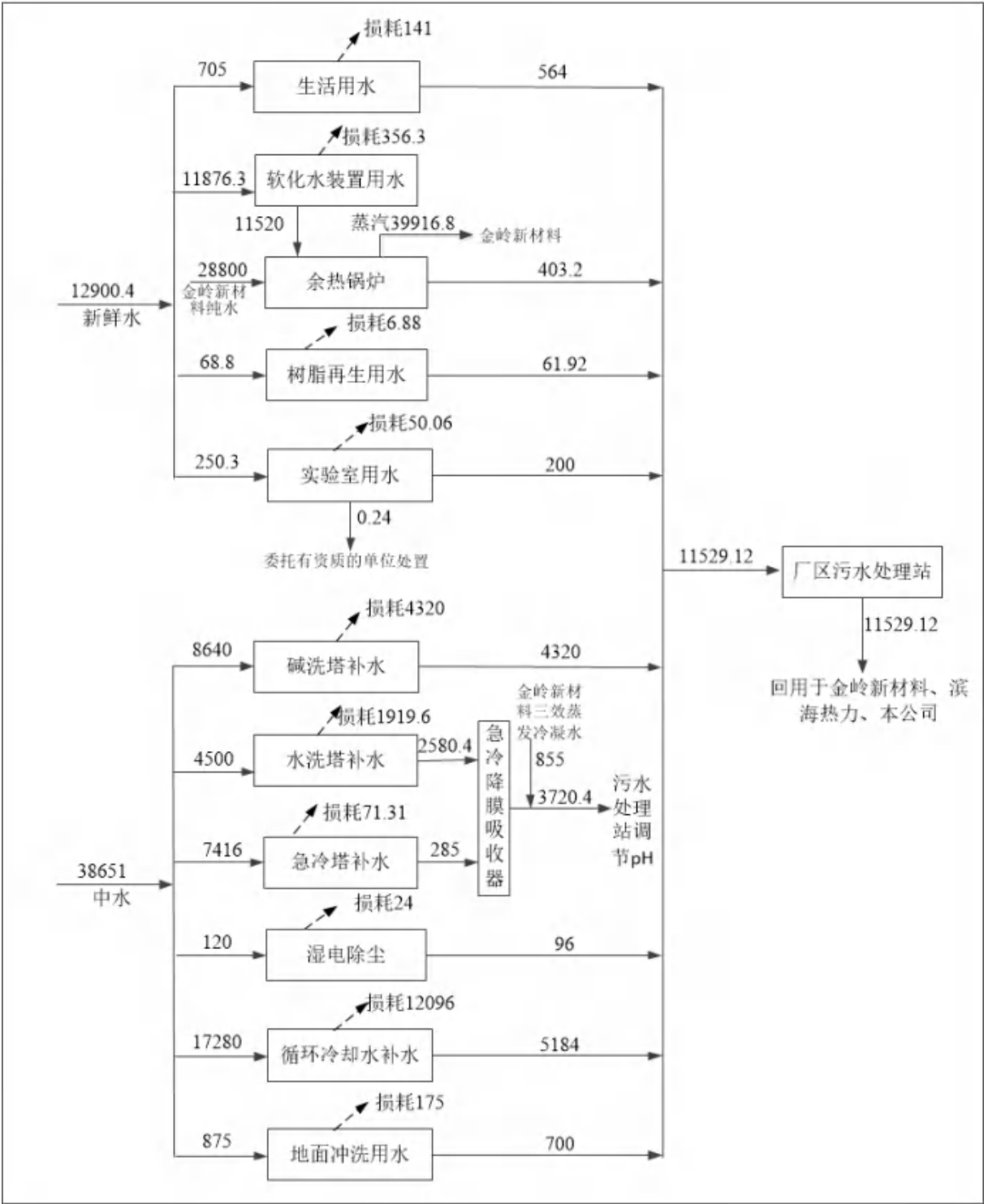
图 4.6-1 水平衡图 (单位: m³/a)
